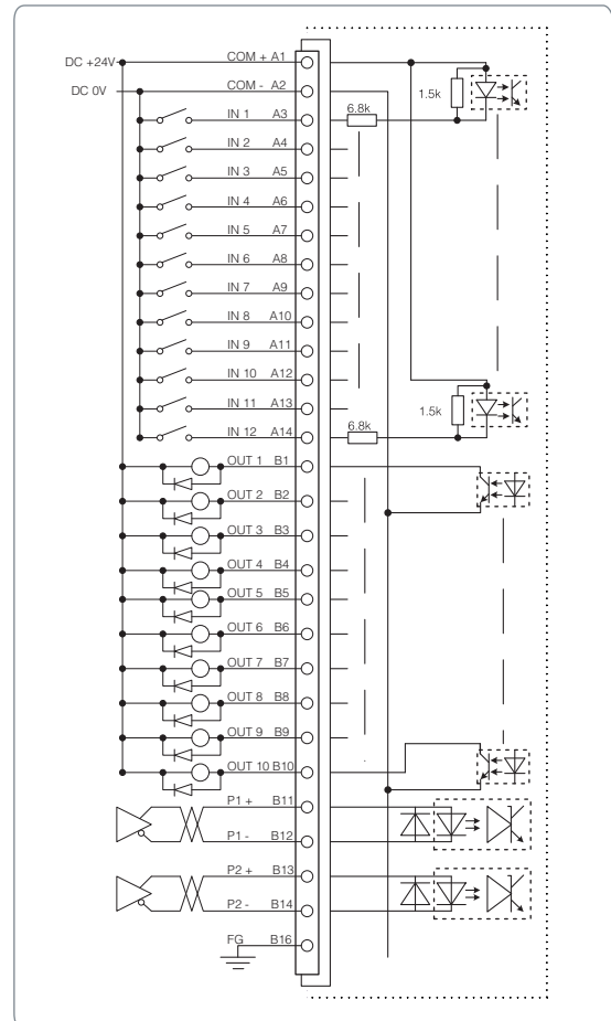
輸入電路 Input Circuit
