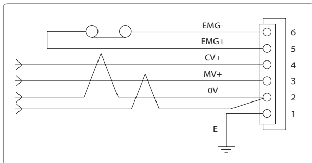
輸入電路 Input Circuit
