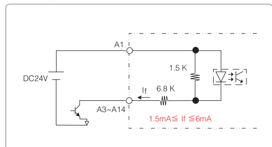
輸出電路 Output Circuit
